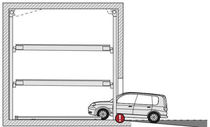
max. 5% Steigung
